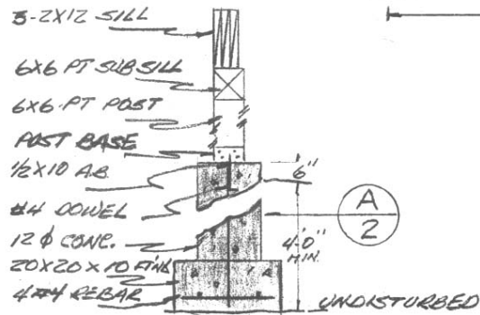
FT'NG / POST / SILL DET. SCALE: 1/2" = 1'-0"
